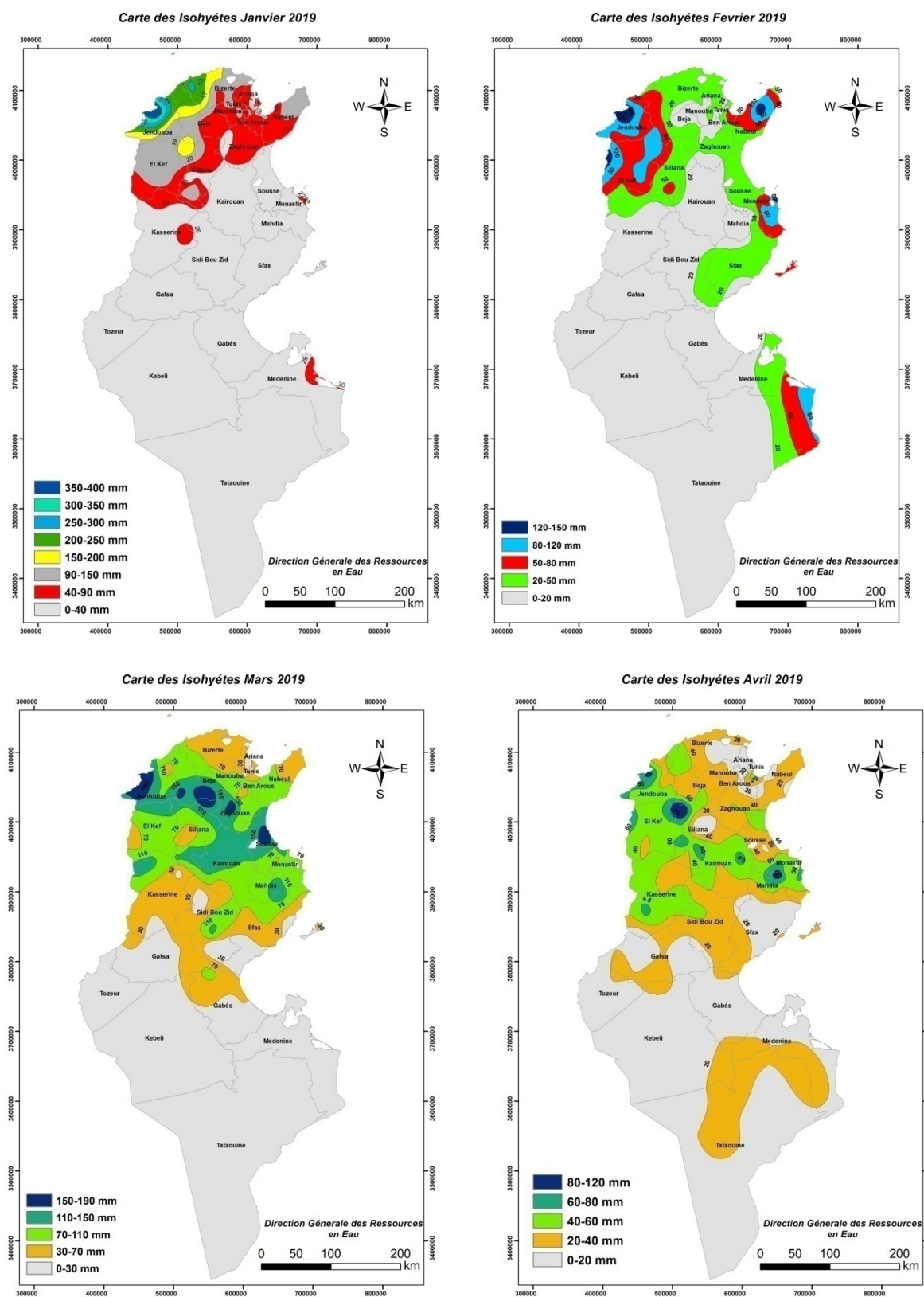
Figure 12 : Isohyètes des pluies mensuelles des mois de (Janv., Fév., Mars et Avril), année 2019
