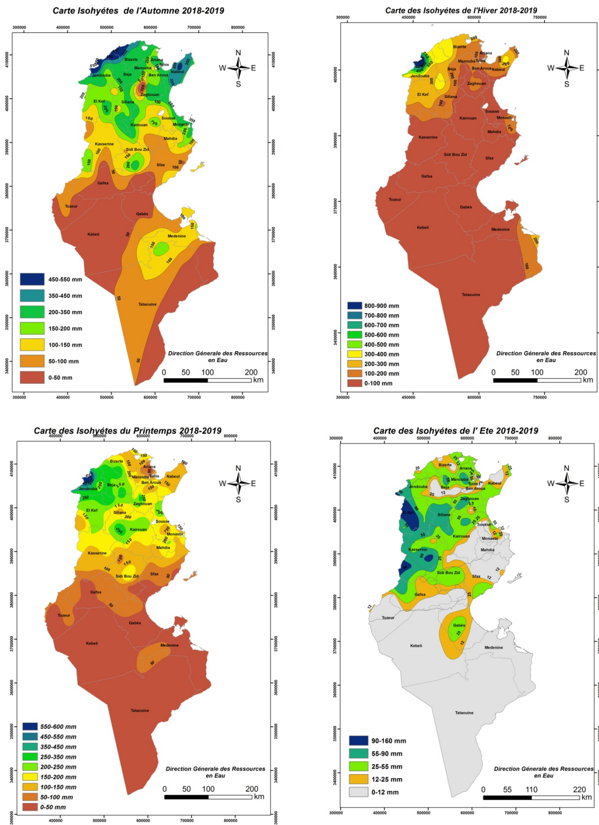
Figure 10: Isohyètes saisonnières de l'année 2018-2019
