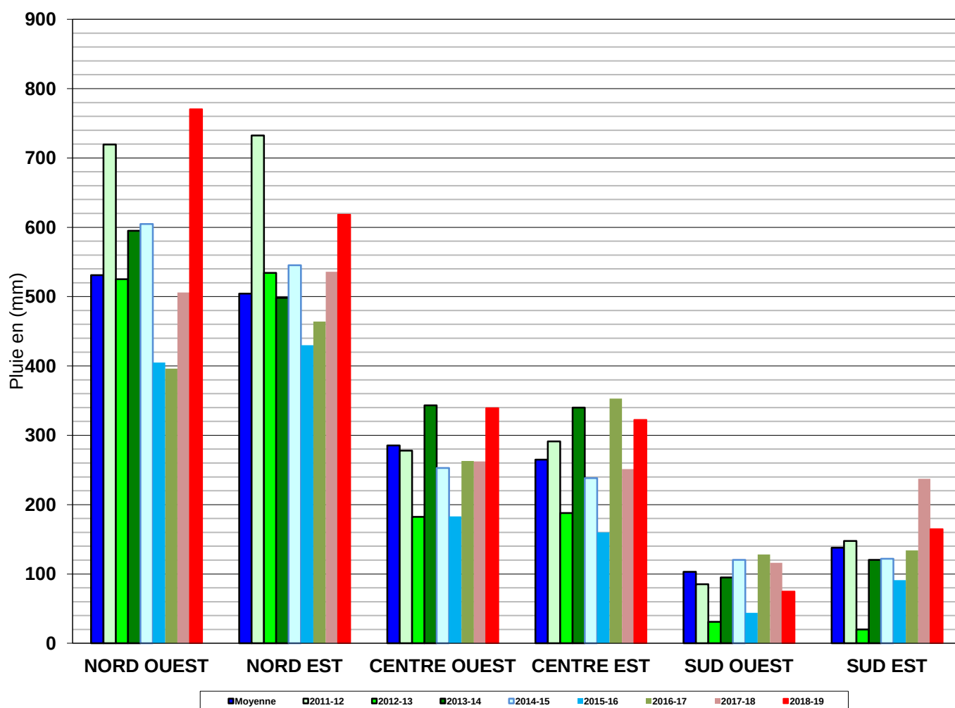
Figure 1 : Comparaison des pluviométries régionales des huit dernières années
