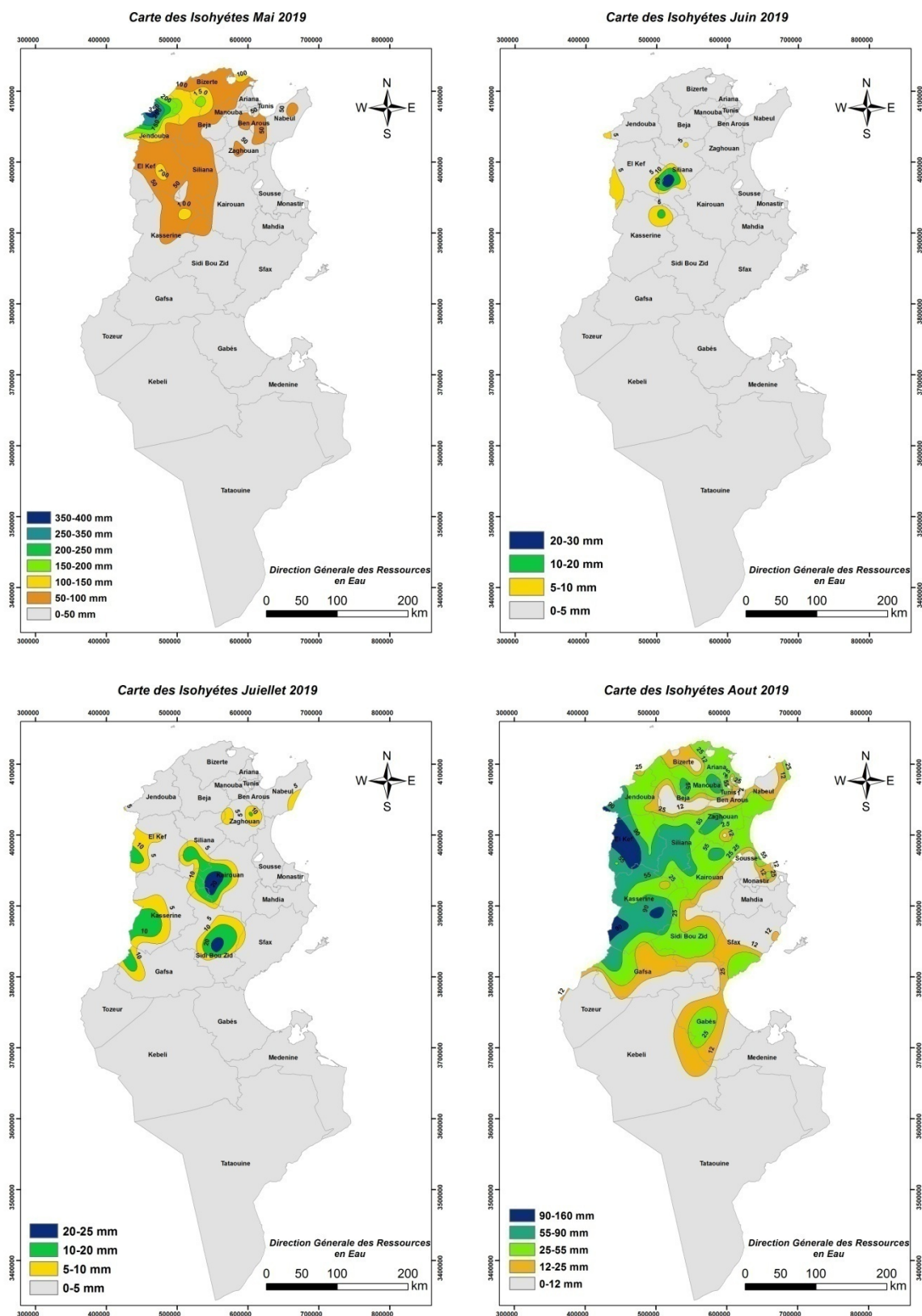
Figure 13: Isohyètes des pluies mensuelles des mois de (Mai, Juin Juil. et Août), année 2019
