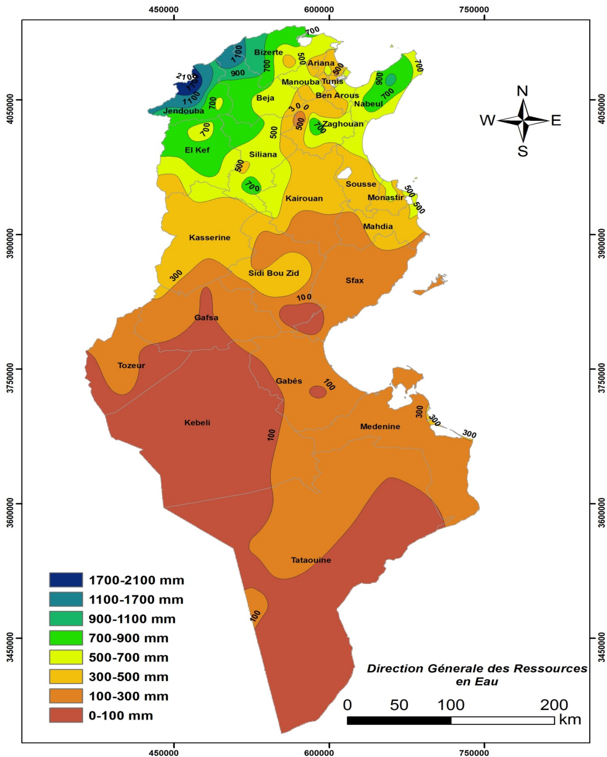
Figure 4 : Isohyètes de l'année 2018-2019
