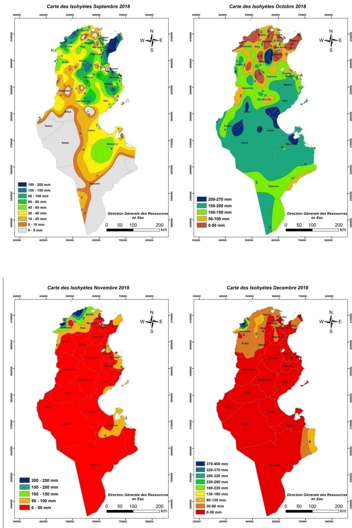
Figure 11: Isohyètes des pluies mensuelles des mois de (Sept., Oct., Nov. et Déc.) année 2018
